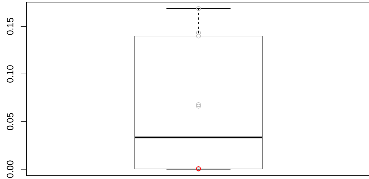
MSE: 0.0587217370795133
