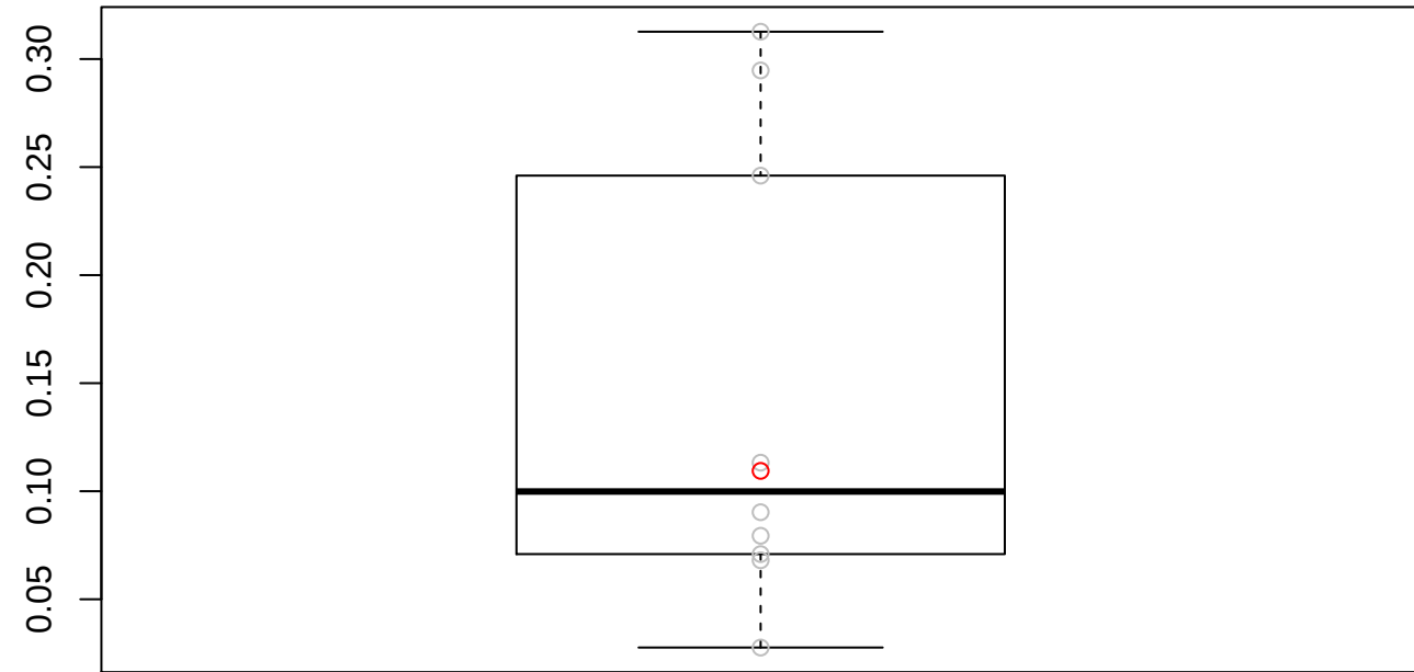
MSE: 0.1412324519746
