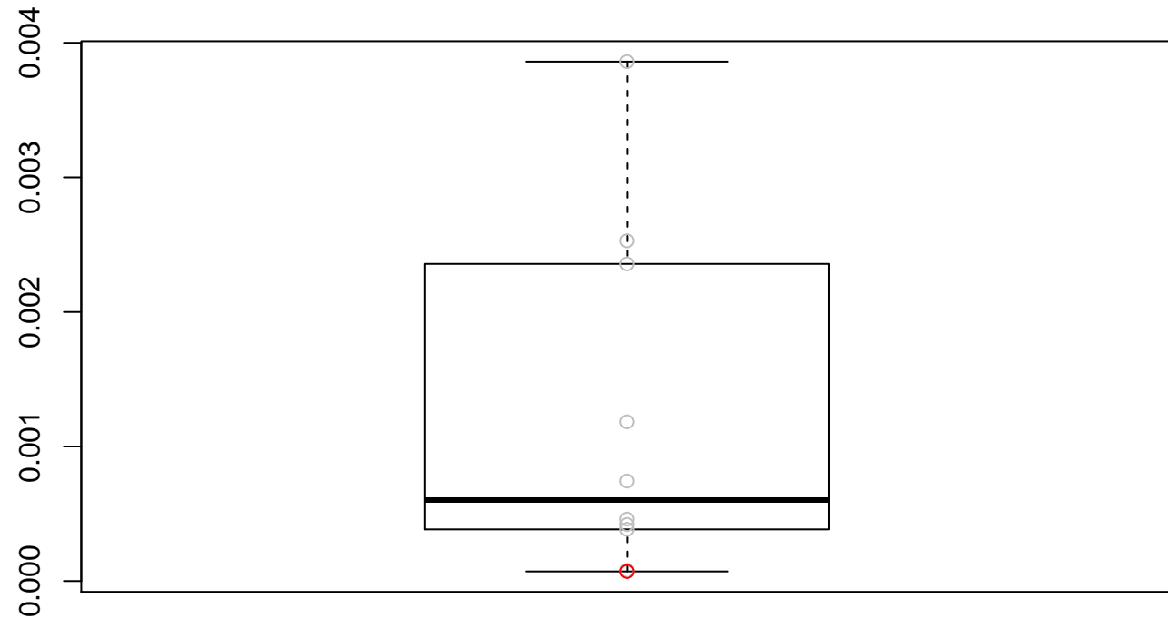
MSE: 0.00120894344161394
