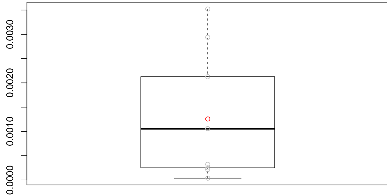
MSE: 0.00127829256433143
