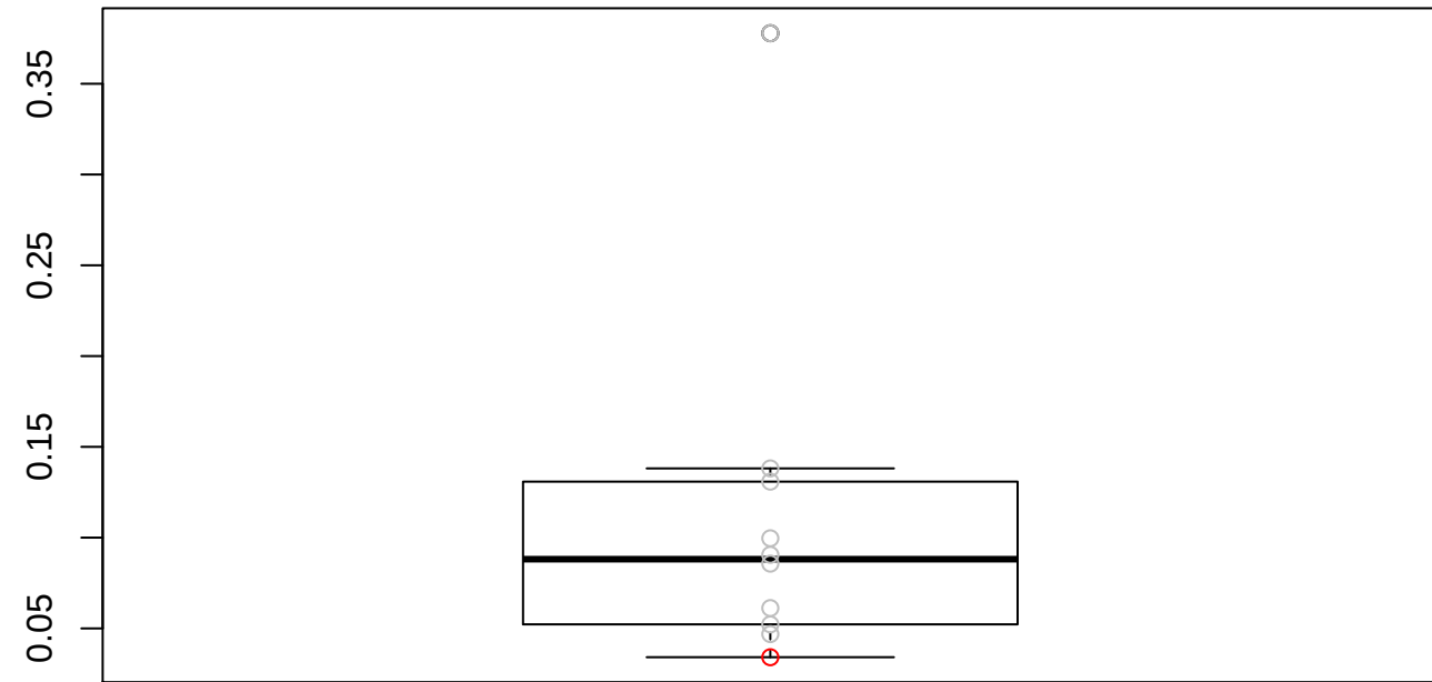
MSE: 0.111714962336433
