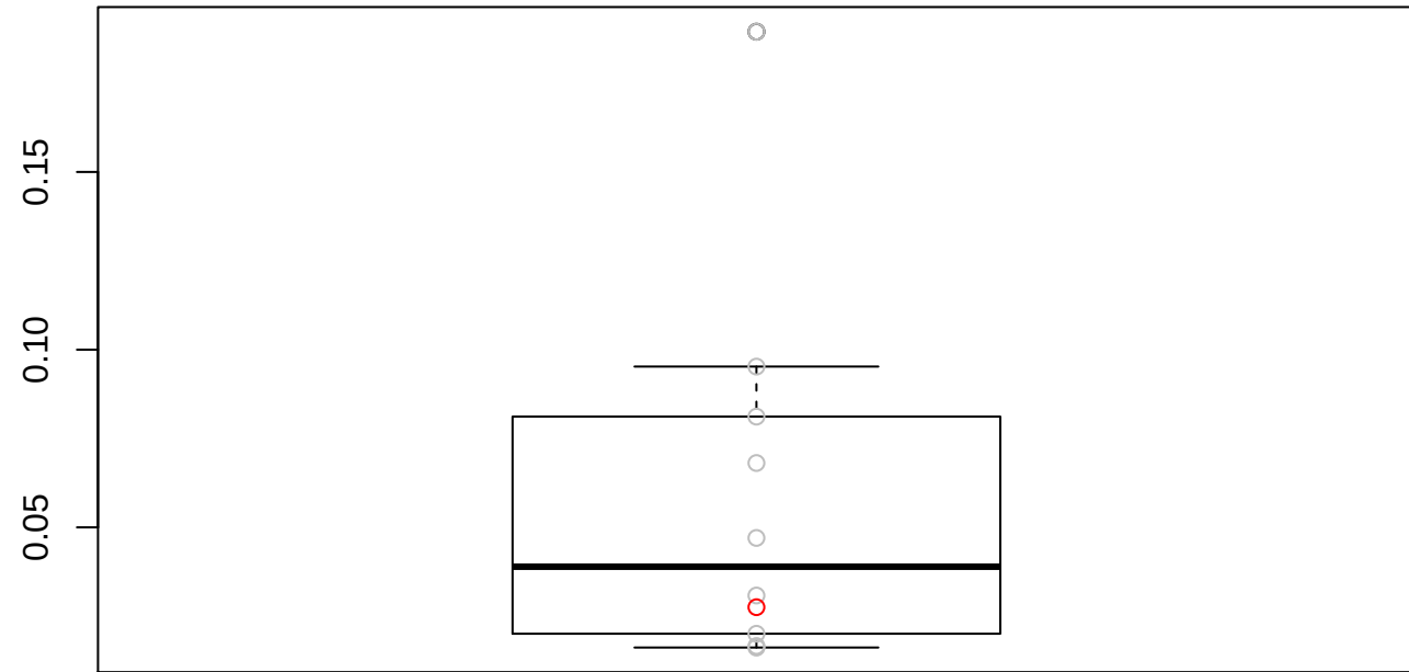
MSE: 0.0592263002239215
