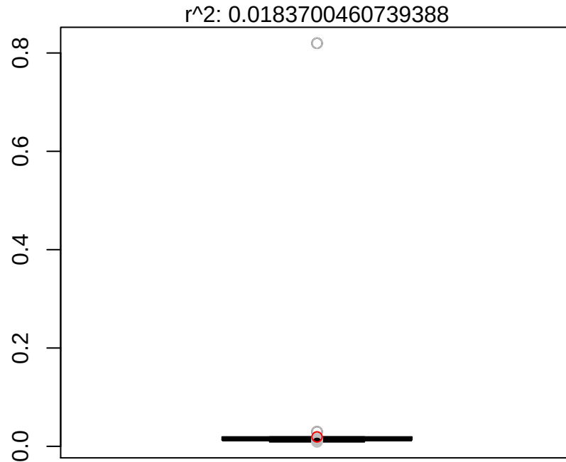
MSE: 0.0960665019879007
