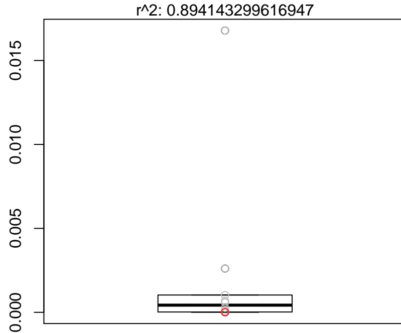
MSE: 0.00220870081937693
