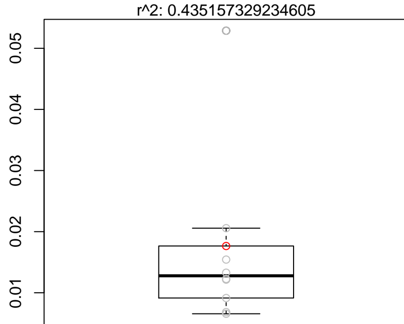
MSE: 0.0166805535797947
