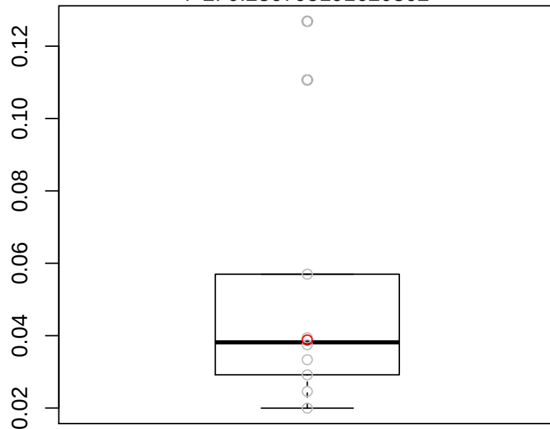
MSE: 0.0517342117989717
