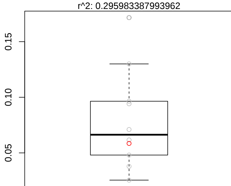
MSE: 0.0794874417164262
