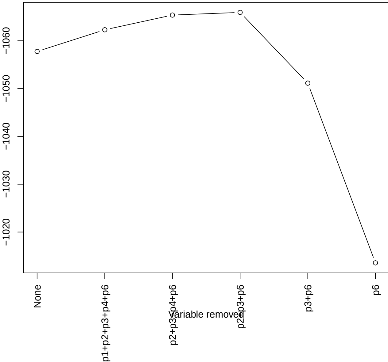
AIC v. variables (UM)
